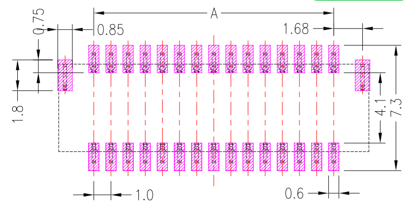
P.C.B LAYOUT
