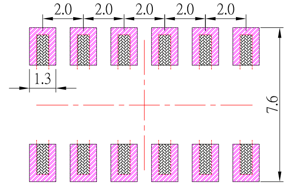
P.C.B LATOUT
