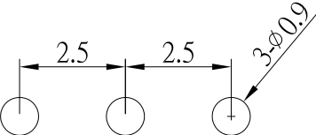
P.C.B LAND PATTERN
