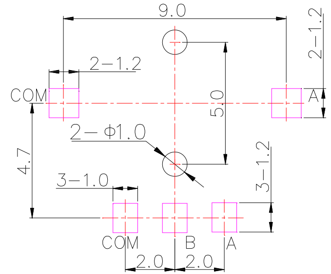
P.C.B LAYOUT
