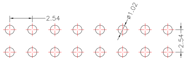
P.C.B. LAYOUT
