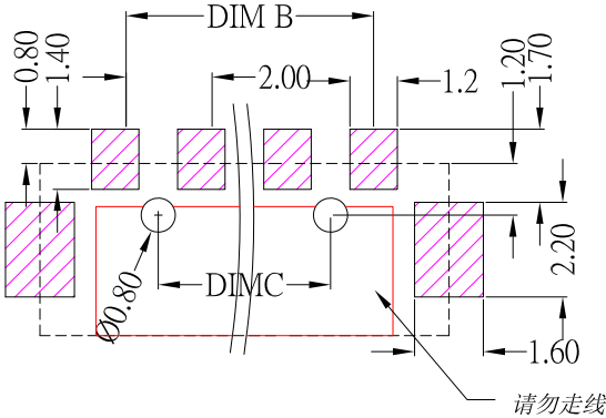
P.C.B LAYOUT
