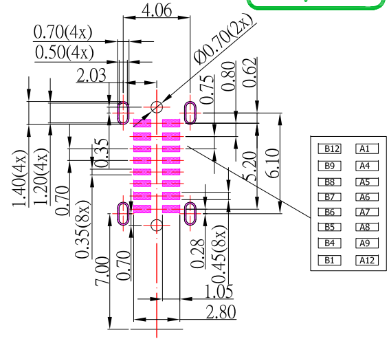
P.C.B. LAYOUT
