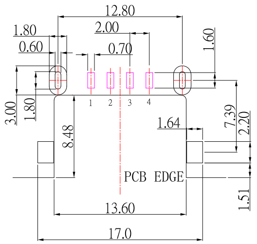
P.C.B LAYOUT
