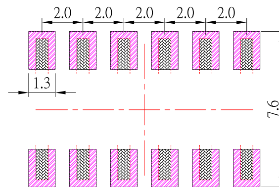
P.C.B LATOUT
