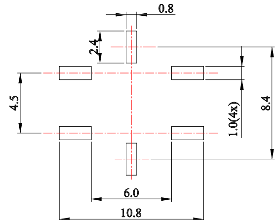
P.C.B LAYOUT
