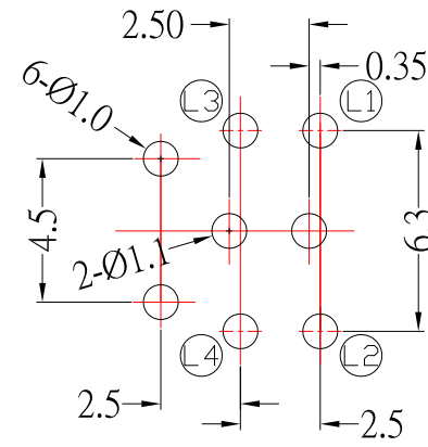
P.C.B LAYOUT
