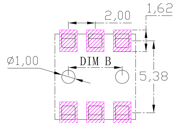
P.C.B LAYOUT
