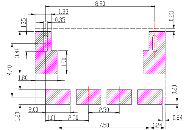
P.C.B LAYOUT
