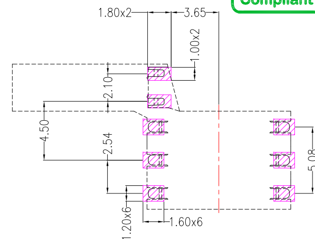
P.C.B Layout
