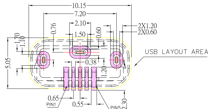
P.C.B LAYOUT
