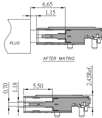
剖面图 比例1:1 A-A
