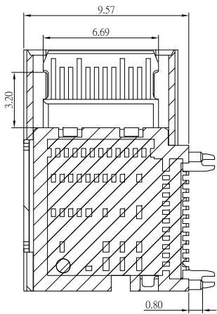
剖視圖
