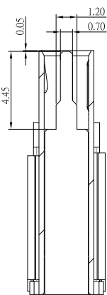
剖視圖
