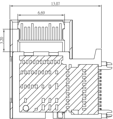
剖視圖
