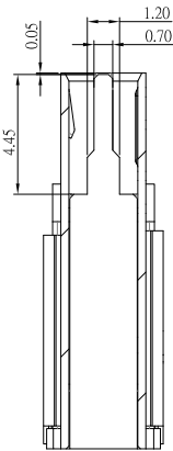
剖視圖
