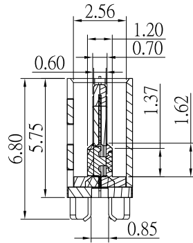
截面 A-A
