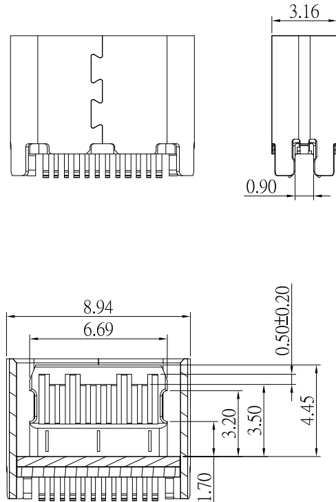
截面 1-1
