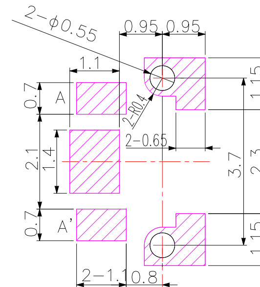
P.C.B LAND PATTERN & HOLE
