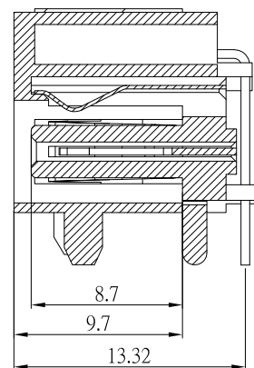
SEC A-A
