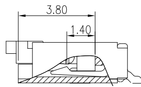
CABLE INSERT DIM. SECTION: A-A
