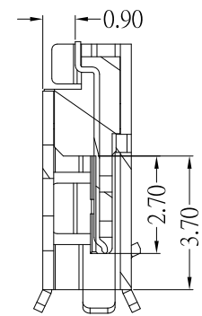
剖面 A-A
