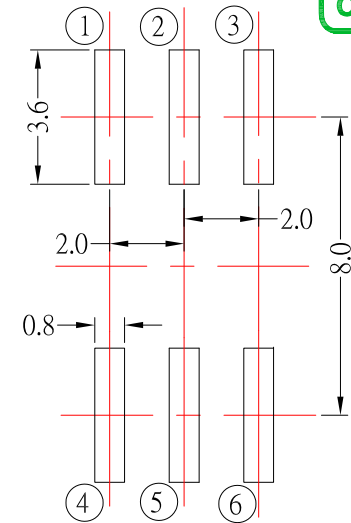
P.C.B LAYOUT
