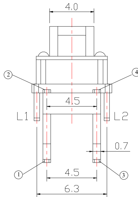
P.C.B LAYOUT
