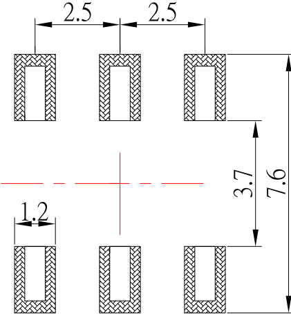
P.C.B LAND PATTERN
