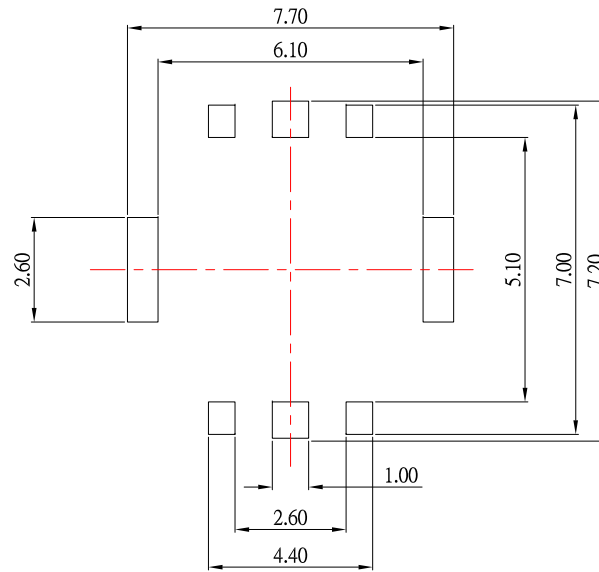
P.C.B LAYOUT
