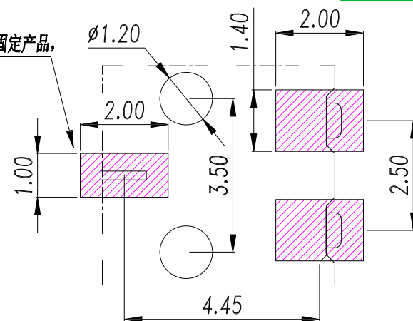
P.C.B LAYOUT
