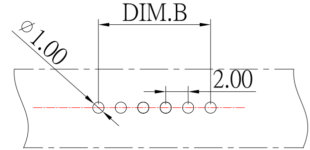
P.C.B LAYOUT
