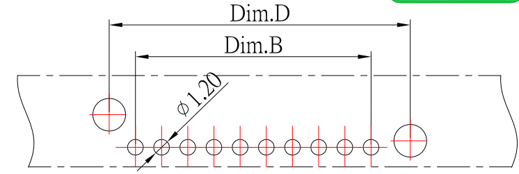
P.C.B LAYOUT
