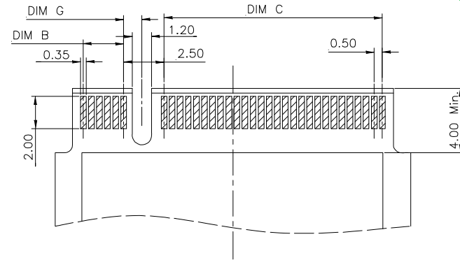
TOP SIDE
