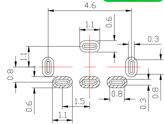
P.B.C LAYOUT
