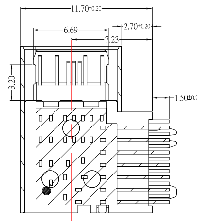
截面 3-3
