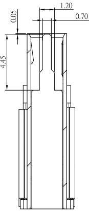
剖視圖
