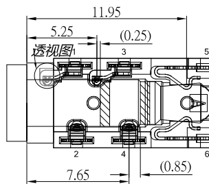
3 级插头接触点位置尺寸
