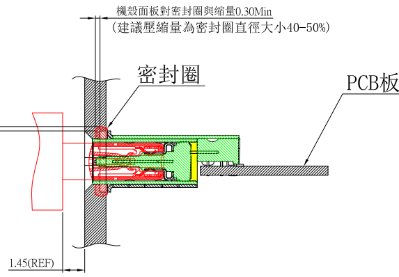
組裝面板後公母頭對插示意圖
