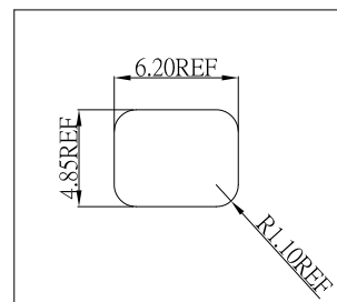
面板開孔參考尺寸
