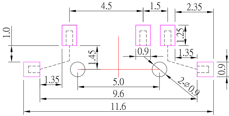
P.C.B LAND PATTERN
