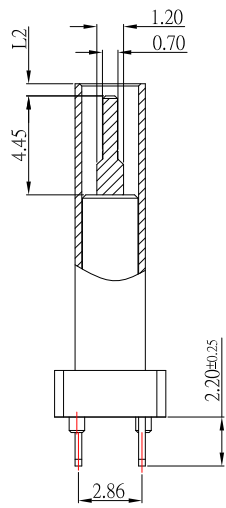
剖視圖
