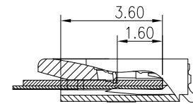
CABLE INSERT DIM.
