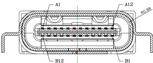
SECTION C-C SCALE: 2:1
