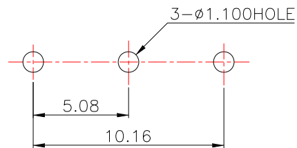
PCB LAYOUT(PATTERN SIDE)
