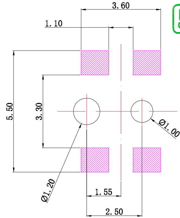
P.C.B LAYOUT
