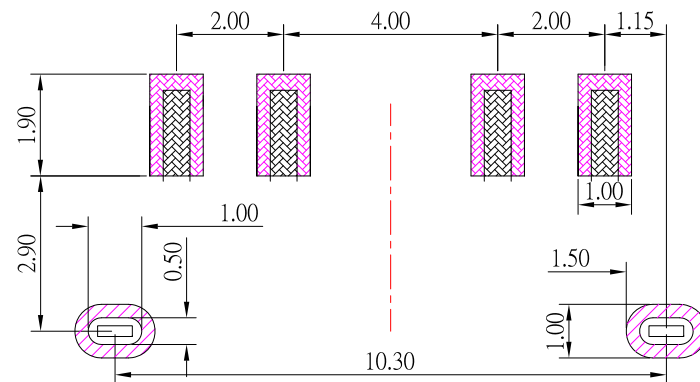
P.C.B LAND PATTERN
